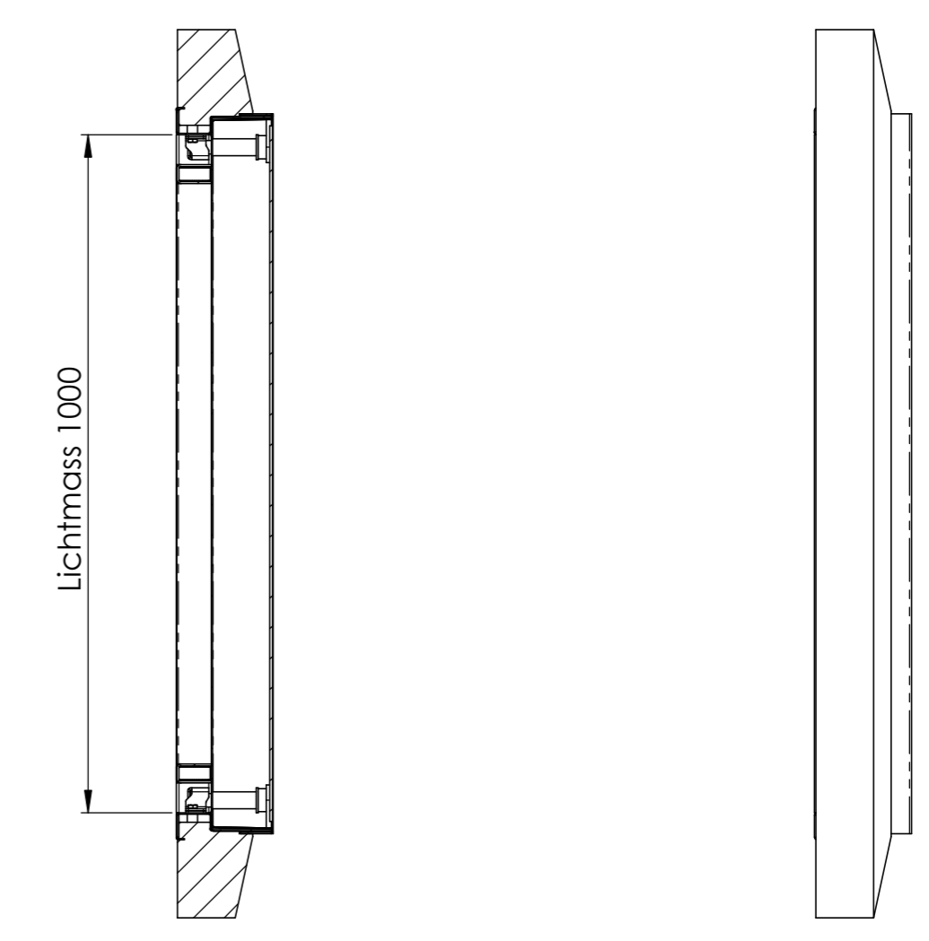
SCHNITT B-B
